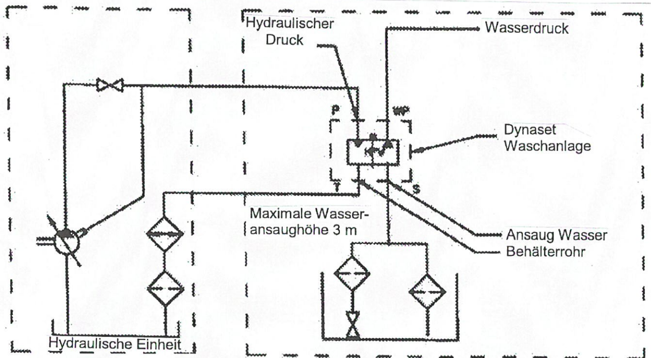
Pumpensystem mit variablen Hubvolumen
