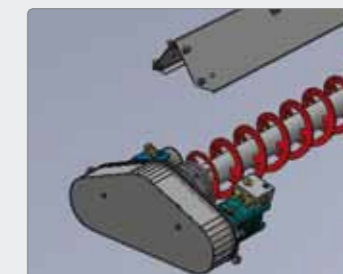
Automatgear med 2 trin. Dette sikrer højt moment ved start af spredning.
