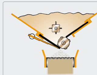
Epoke-princippet sikrer, at udlægning af alle former for spredematerialer sker ensartet og nøjagtigt uanset temperaturforhold og materialets beskaffenhed.
