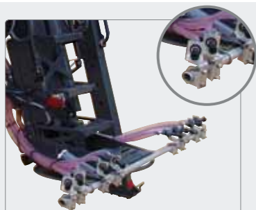
Højhastigheds-spredning med Spratronic-dyser. Spredner effektivt ved hastigheder op til 90 km/t.
